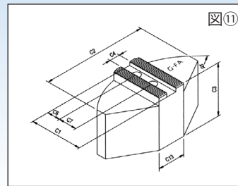
円形生爪
